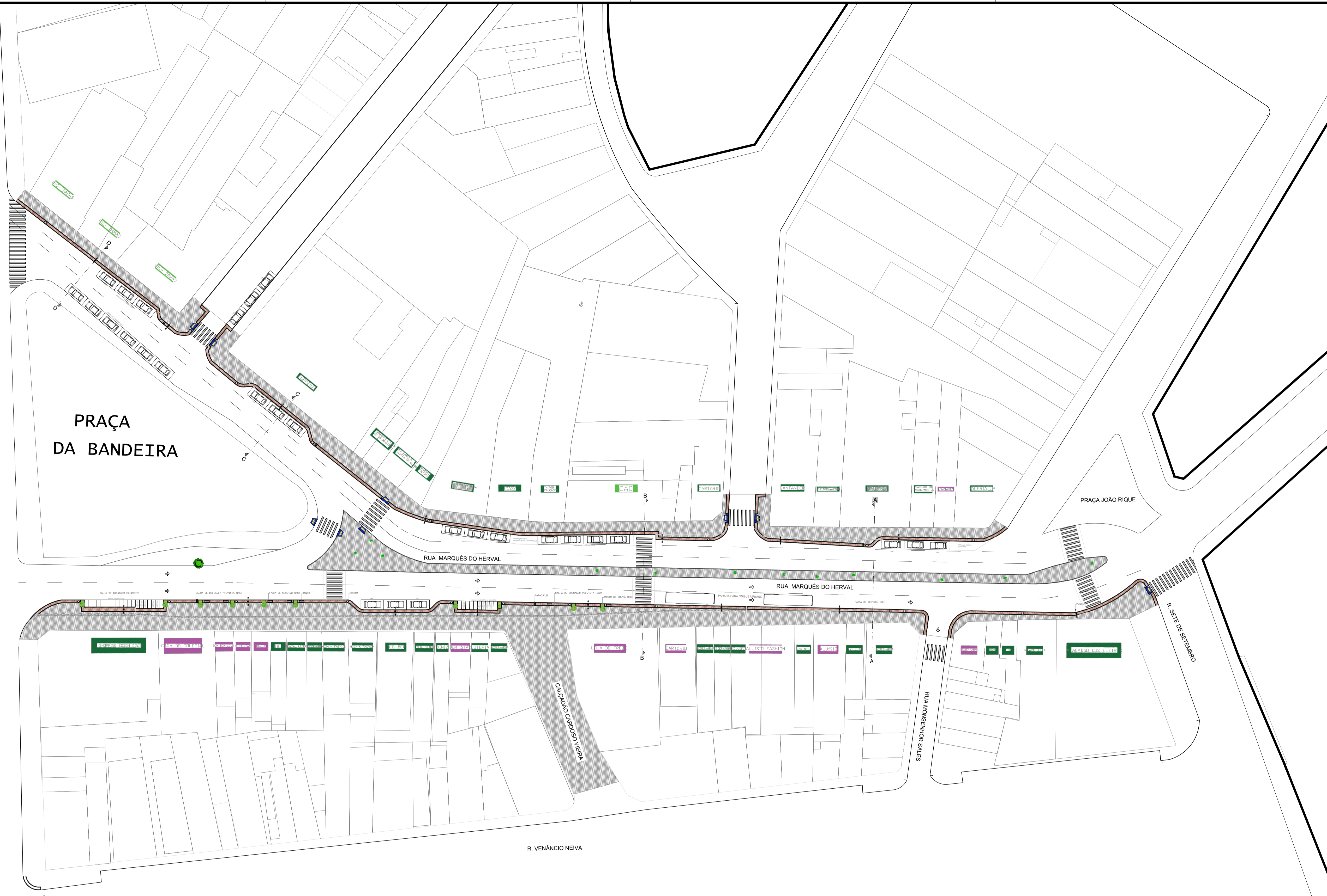
PLANTA BAIXA PROPOSTA ESCALA 1:500
